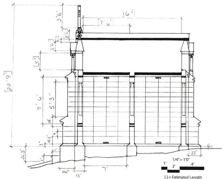
Right Elevation
